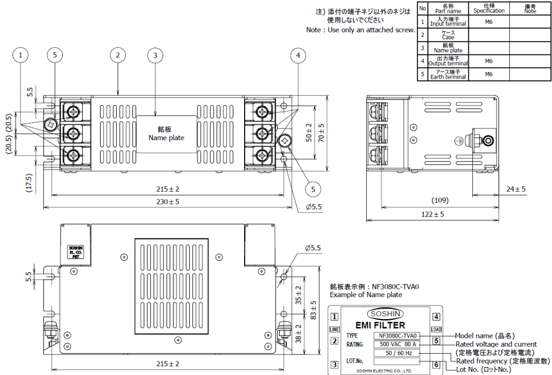
fig.2 NF3000C-TVA0(80~100A)
