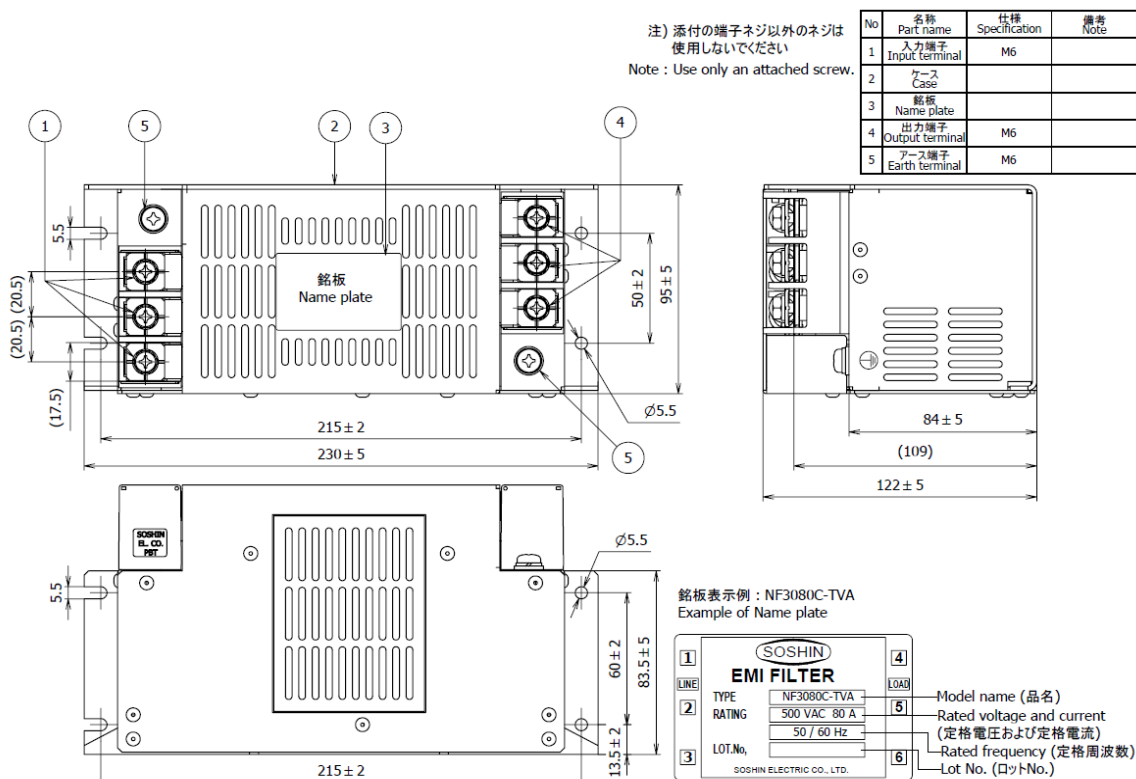
fig.1 (80~100A)
